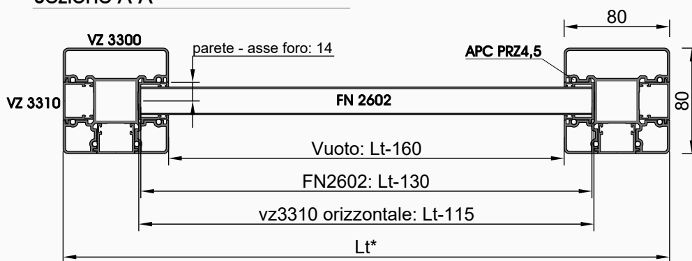
Sezione A-A
